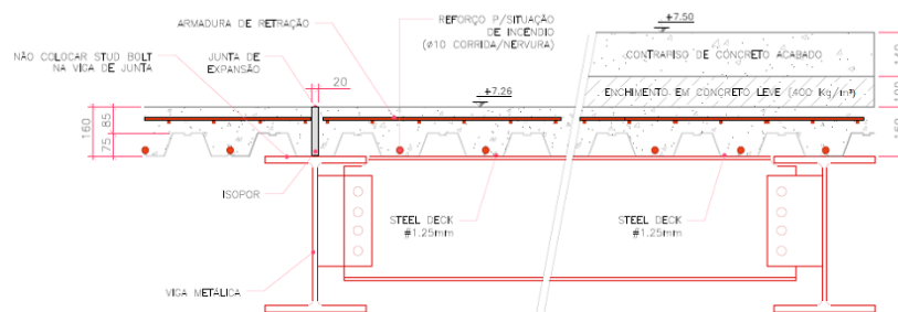
(B) DETALHE TÍPICO DAS LAJES ESC. 1:10
