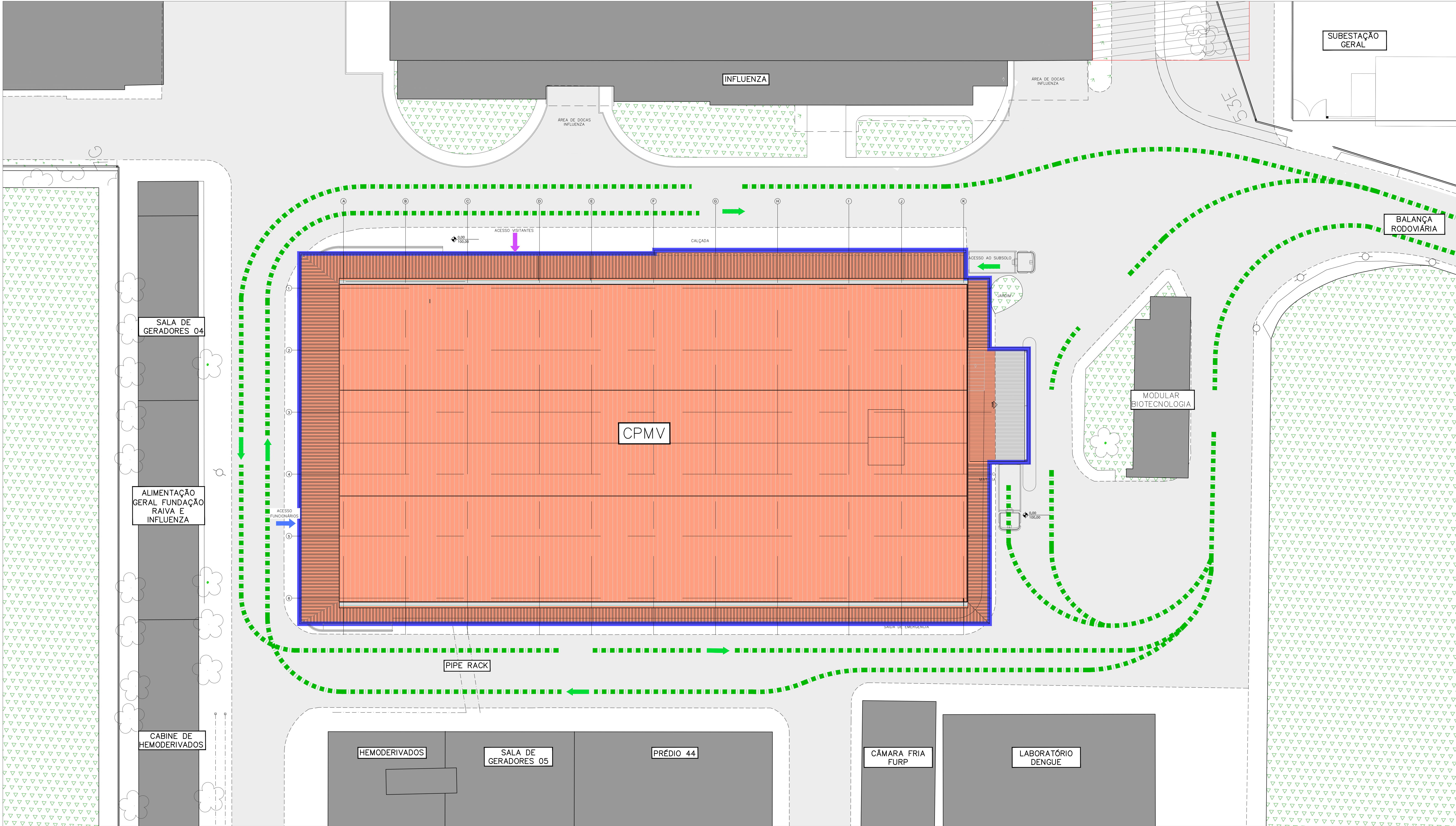
NP 01 IMPLANTAÇÃO 00044 1/200
