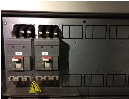
Foto 2 - Espaço disponível para instalação do novo disjuntor - Vista Interna.
